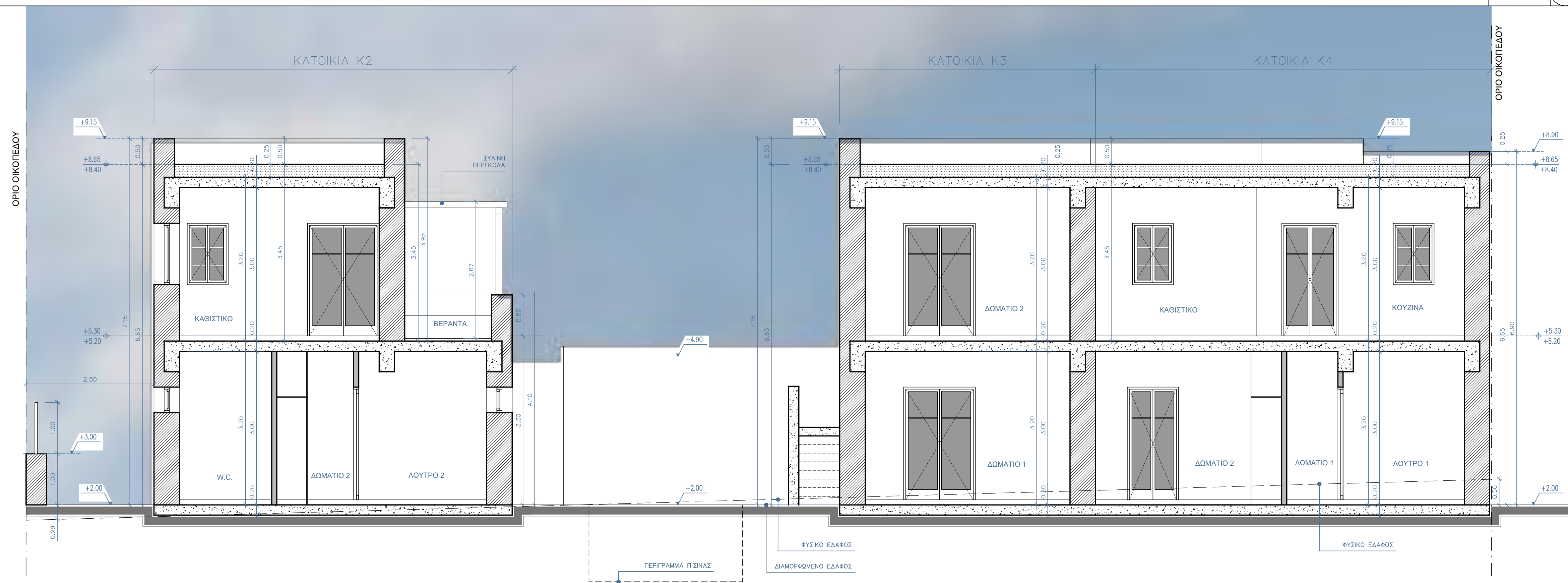
ΤΟΜΗ Γ-Γ
